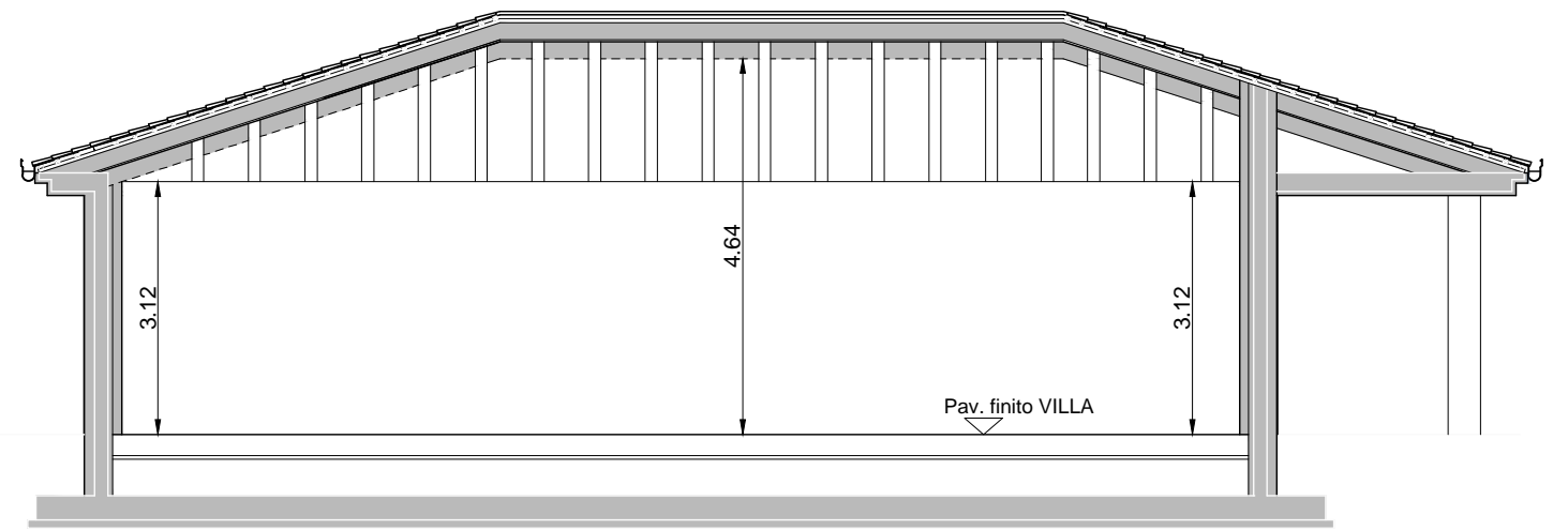
SEZIONE LONGITUDINALE A - A
