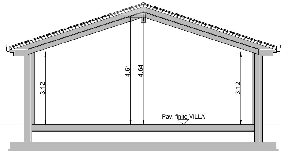
SEZIONE TRASVERSALE B - B
